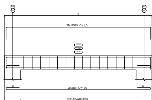
DETALHE VIGA
