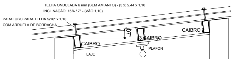
CORTE AA Sem escala
