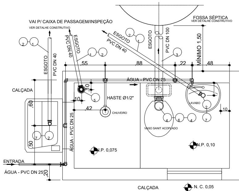
PLANTA - INSTALAÇÃO HIDROSSANITÁRIA
