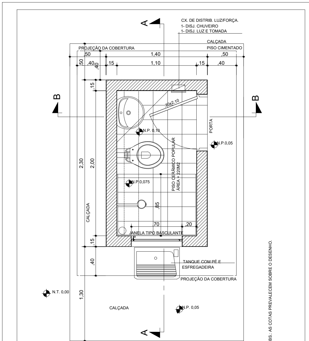
PLANTA BAIXA
