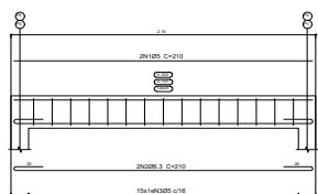
DETALHE VIGA
