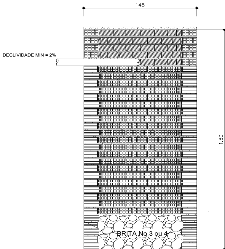
SUMIDOURO CORTE FF
